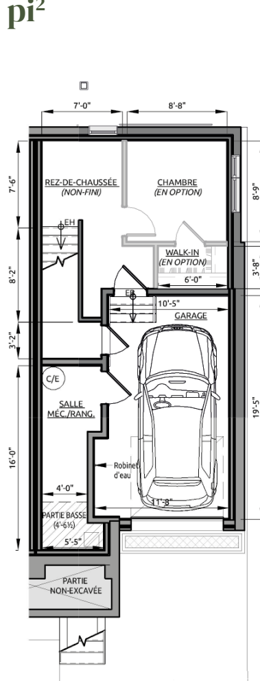
Étage 1 - 292 pi 2 + garage 362 pi 2
