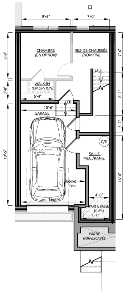
Étage 1 - 297 pi 2 + garage 355 pi 2
